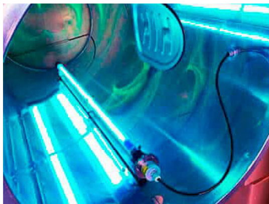
Instalación de generadores de UV-C en los conductos; si es necesario se instalan tapas de registro para facilitar el montaje y el mantenimiento.
